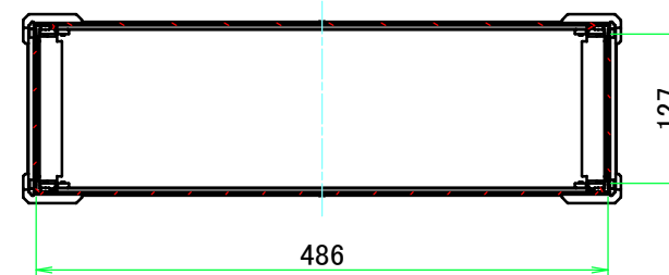
A-A (1:7)
