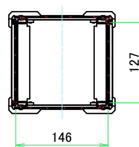
A-A (1:6)
