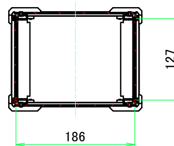
A-A (1:6)
