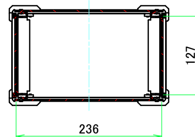
A-A (1:6)
