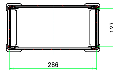
A-A (1:6.5)
