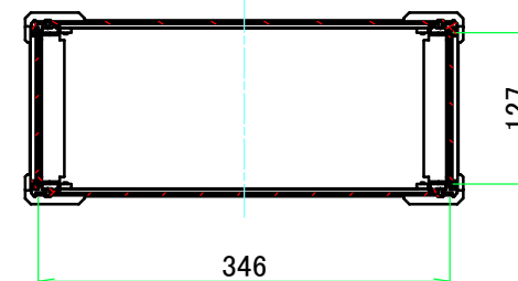
A-A (1:7)
