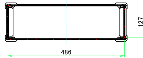
A-A (1:8)
