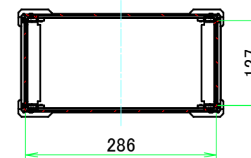
A-A (1:8)
