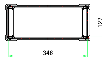
A-A (1:8)
