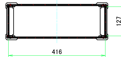
A-A (1:8)
