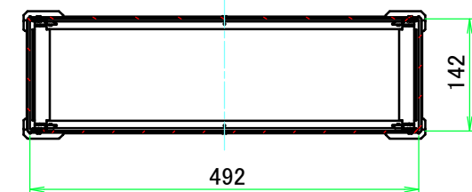
C-C ( 1 : 8.5 )
