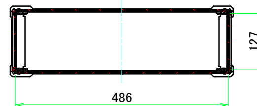
A-A ( 1 : 8.5 )
