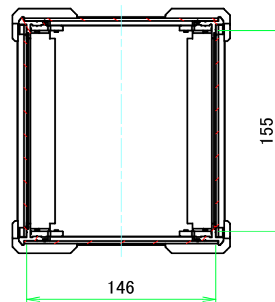
A-A ( 1 : 4 )
