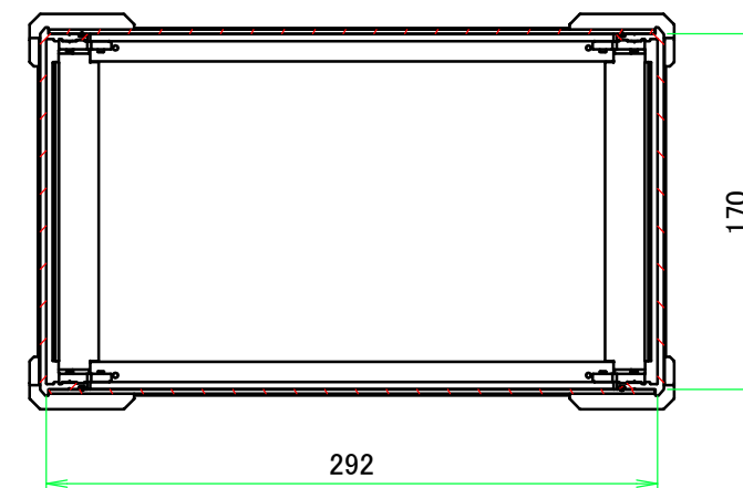
C-C ( 1 : 4 )
