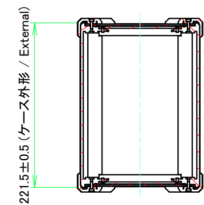
D-D (1:5)
