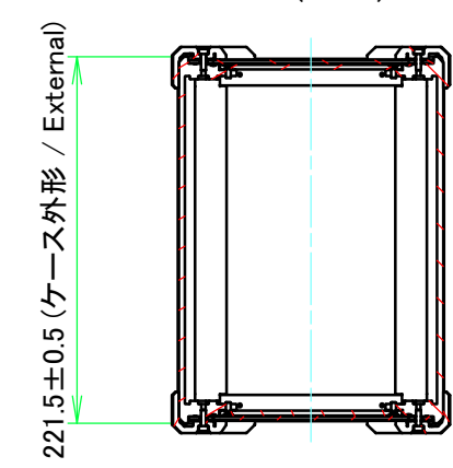
D-D (1:5)
