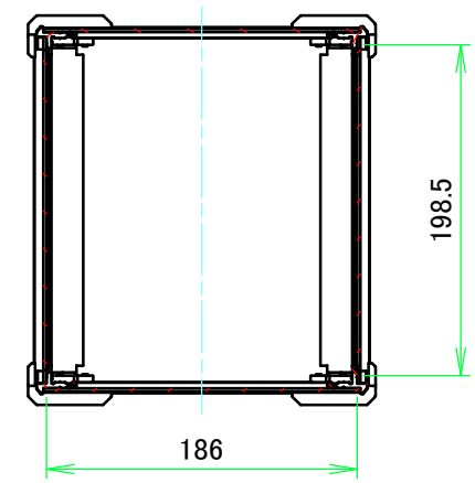
A-A (1:5)
