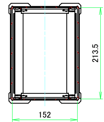
C-C ( 1 : 5.5 )
