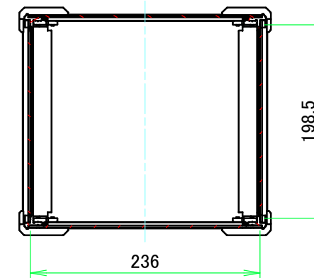
A-A ( 1 : 5.5 )
