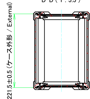
D-D ( 1 : 5.5 )
