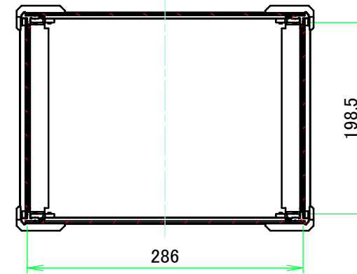
A-A ( 1 : 5.5 )
