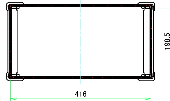
A-A ( 1 : 6.5 )
