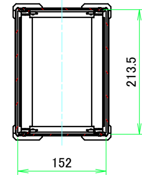
C-C ( 1 : 6.5 )
