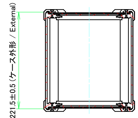
D-D (1:5)
