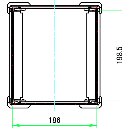
A-A (1:5)
