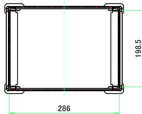
A-A (1:6)
