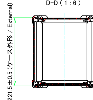
D-D (1:6)
