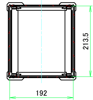
C-C ( 1 : 6.5 )
