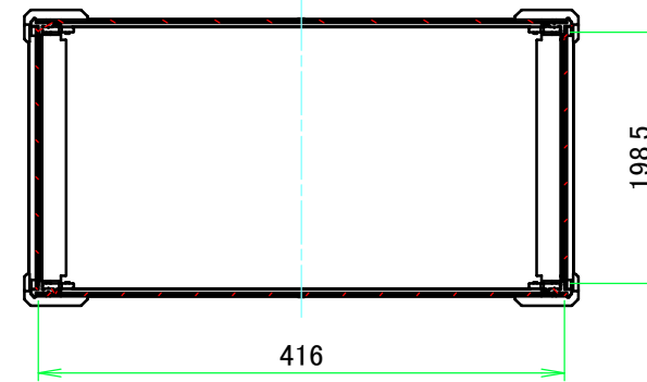
A-A ( 1 : 6.5 )
