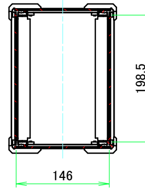
A-A (1:6)
