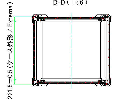
D-D (1:6)
