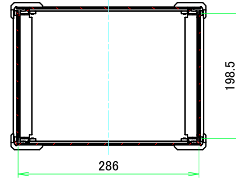
A-A (1:6)
