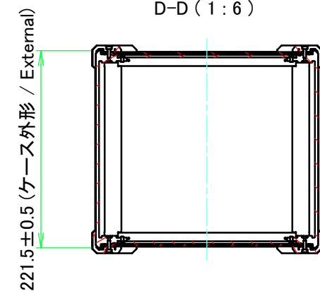
D-D (1:6)
