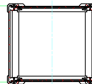
D-D (1:6.5)
