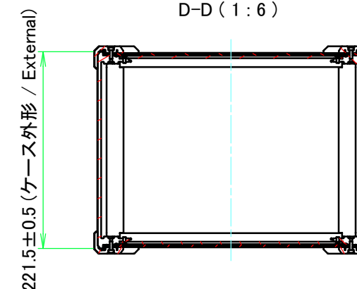
D-D (1:6)
