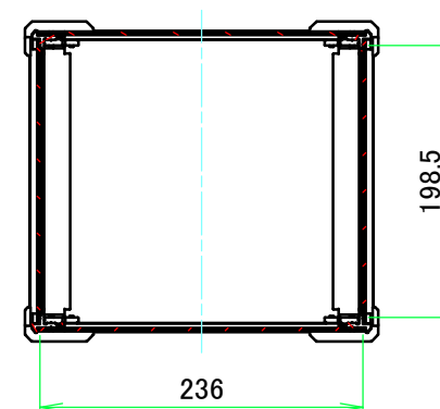
A-A (1:6)
