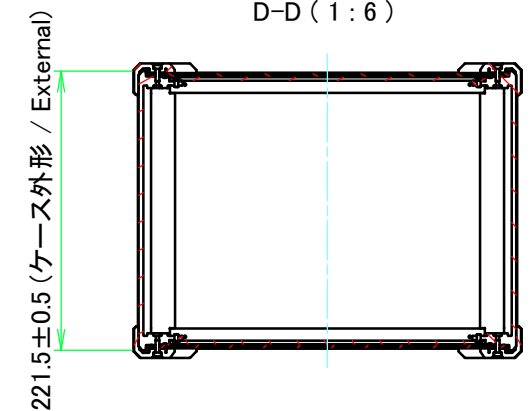
D-D (1:6)
