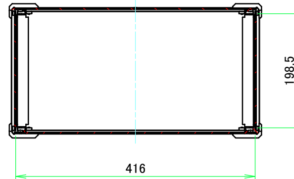
A-A (1:6.5)
