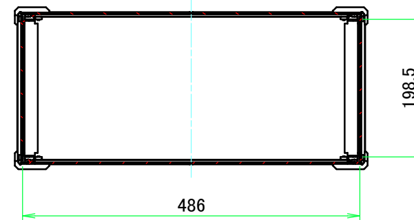
A-A (1:7.5)
