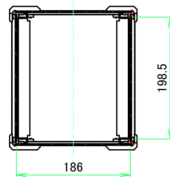
A-A (1:6)
