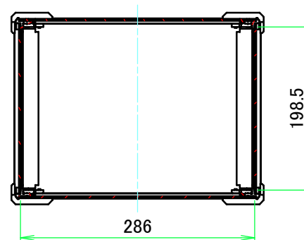
A-A (1:6.5)
