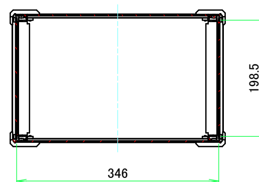
A-A (1:6.5)
