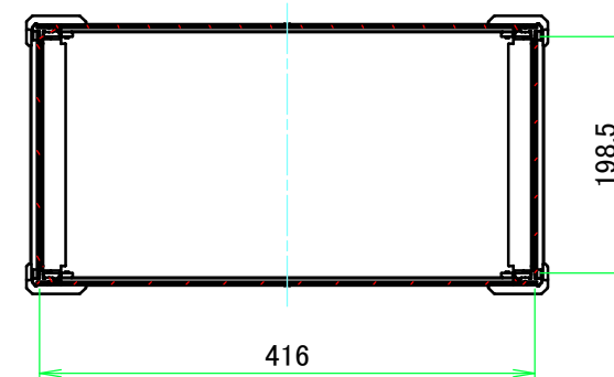
A-A (1:7)
