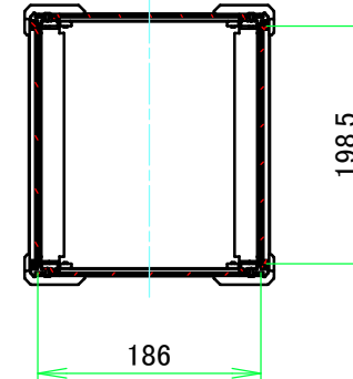
A-A (1:7)
