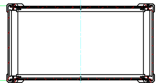
D-D (1:7)
