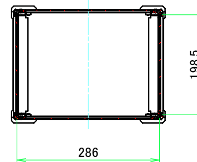
A-A ( 1 : 7.5 )
