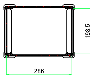
A-A (1:8)
