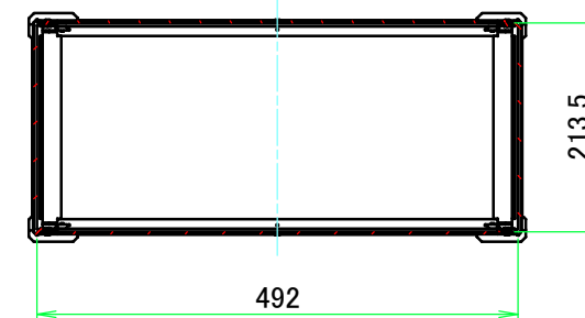
C-C ( 1 : 8.5 )
