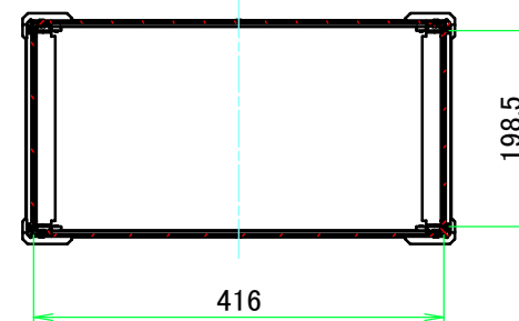
A-A ( 1 : 8.5 )
