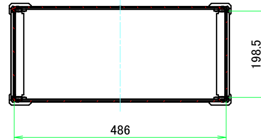
A-A ( 1 : 8.5 )
