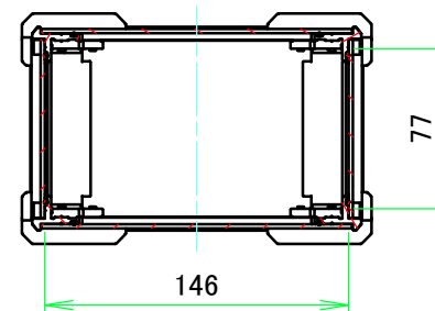
A-A (1:4)
