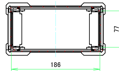
A-A (1:4)
