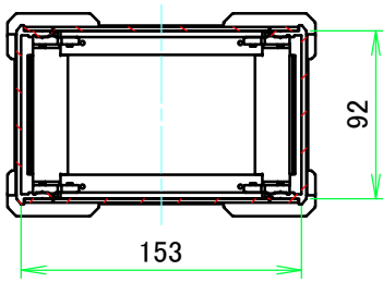
C-C ( 1 : 4.5 )
