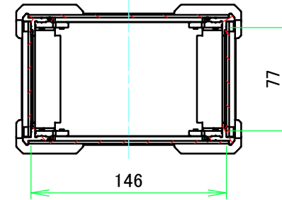
A-A (1:4)
