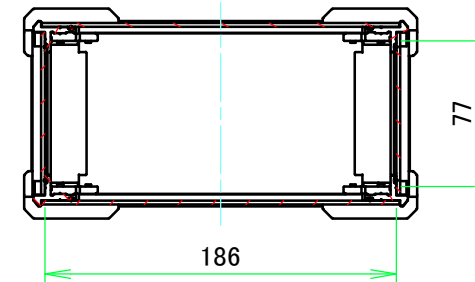
A-A (1:4)
