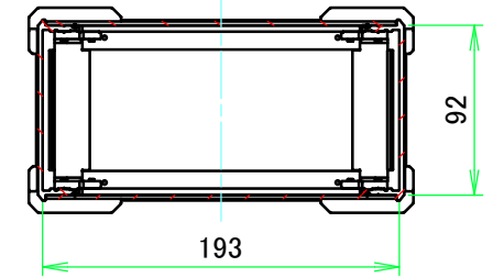
C-C ( 1 : 4.5 )
