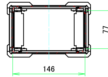
A-A (1:4.5)
