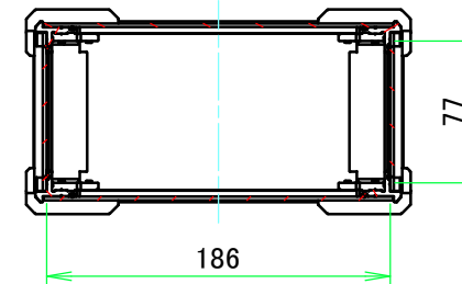
A-A ( 1 : 4.5 )
