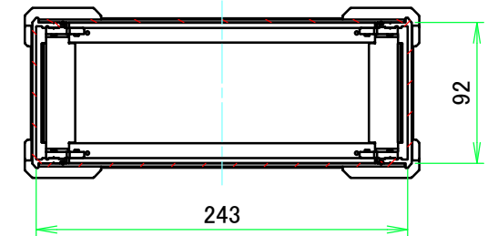
C-C ( 1 : 4.5 )
