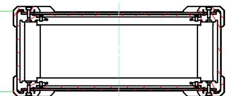
D-D ( 1 : 4.5 )
