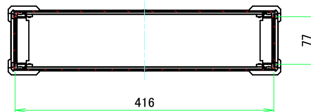
A-A (1:6)
