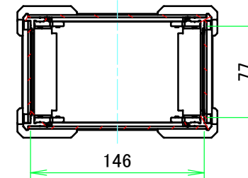
A-A ( 1 : 4.5 )
