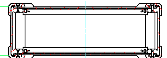
D-D ( 1 : 4.5 )
