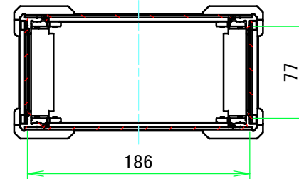
A-A (1:4.5)
