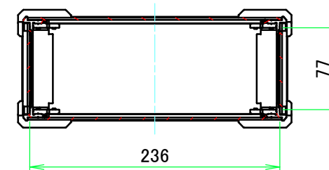
A-A (1:5)
